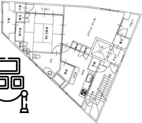
3階平面図
